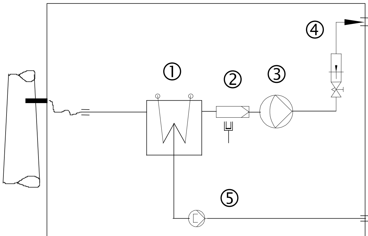
Abbildung 1 Gasflussschema
