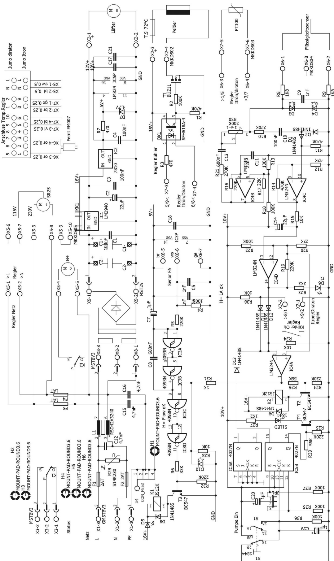
Abbildung 16 Stromlaufplan CSS-M...
