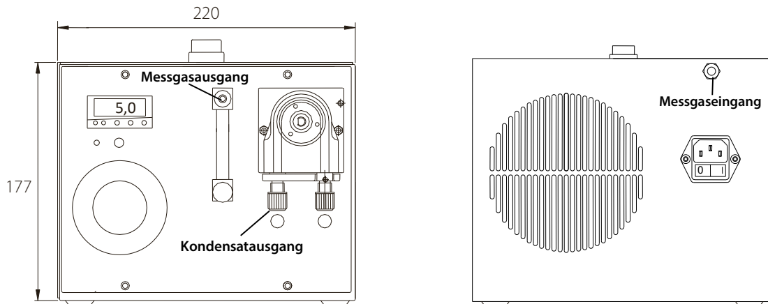
Abbildung 3 Schlauchanschlüsse CSS-M tragbar
