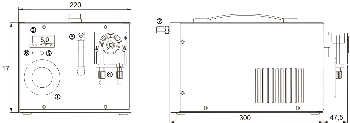
Abbildung 2 Abmessungen CSS-M
